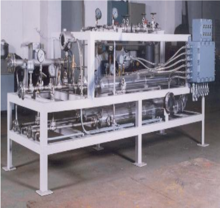
LNG Sampling Vaporizer
